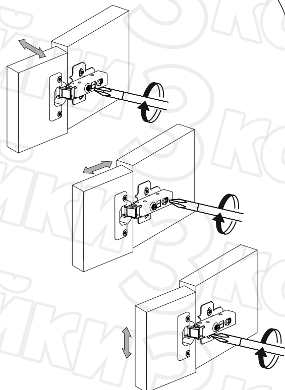
РЕГУЛИРОВКА ФАСАДОВ ДВЕРОК
