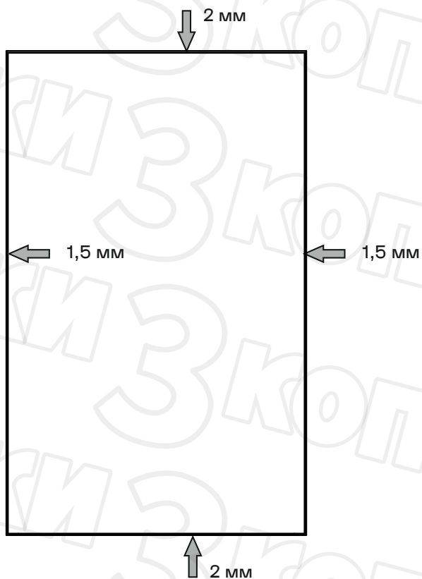
РЕГУЛИРОВКА ФАСАДОВ ДВЕРОК
