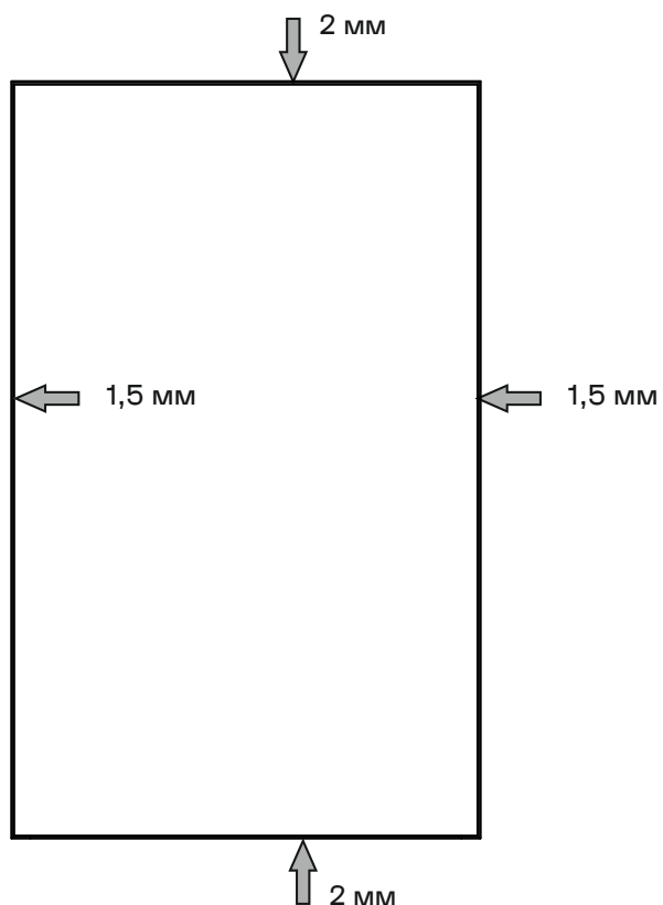
РЕГУЛИРОВКА ФАСАДОВ ДВЕРЕК
